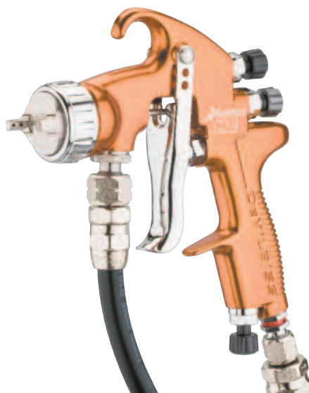
Advance HD Trans-Tech Kesselpistole mit hochwertigen Devilbiss Schläuchen und Anschlüssen
